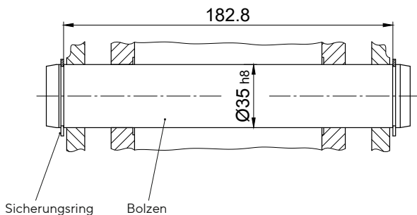
Obere Aufhängung
