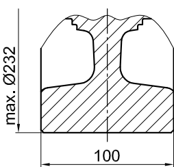
Form 9 ohne Spurkränze
