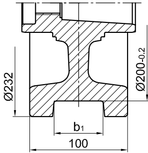
Form 1 beidseitiger Spurkranz
