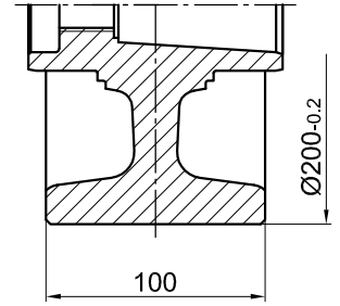
Form 4 ohne Spurkränze mit zylindrischer Lauffläche
